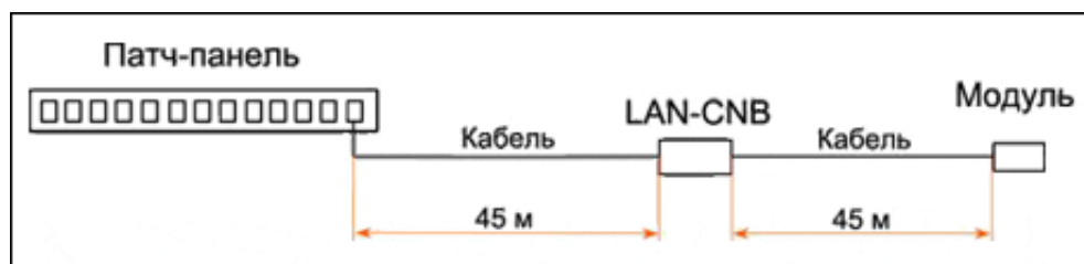
Схема установки консолидационной точки
