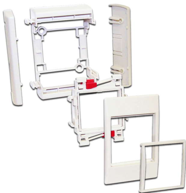
Сборка коробки
