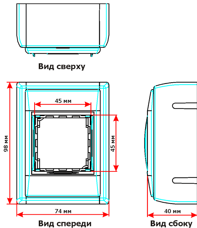
Составные детали
