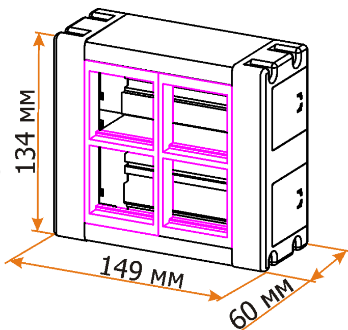
Размеры
