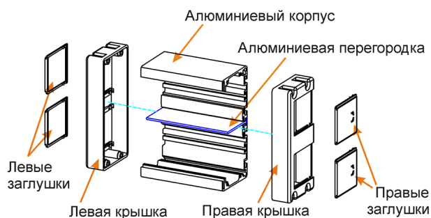
Сборка
