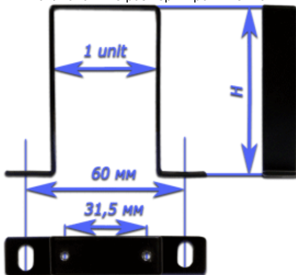
Установочные размеры кронштейнов
